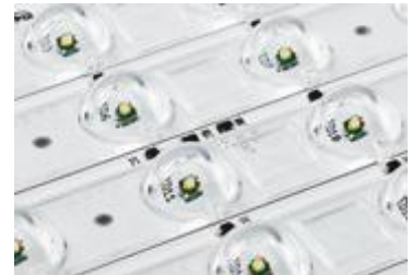
Figuur 7: Voorbeeld 2 PCB met leds en lenzen
