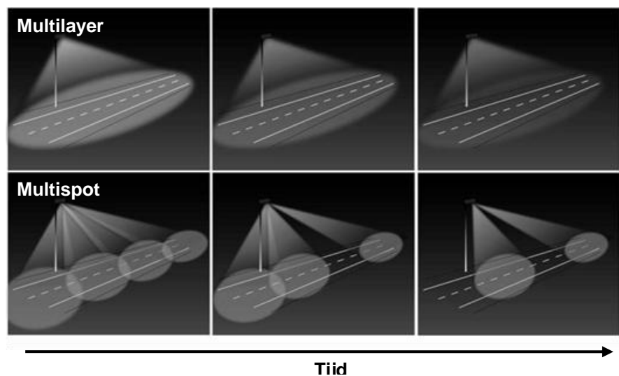
Figuur 9: Verschil tussen Multilayer en Multispot
